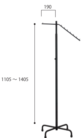
H-2121 - A / B セレクトスロープハンガー
