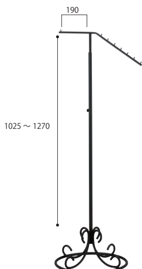
H-2141 スロープハンガーパールA
