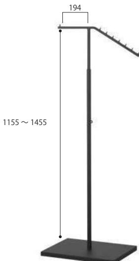
H-2280 NスロープハンガーC
